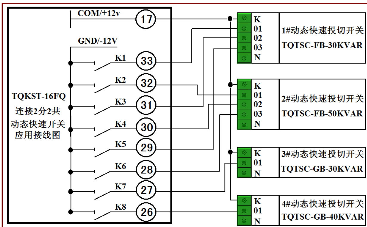
典型应用接线图
